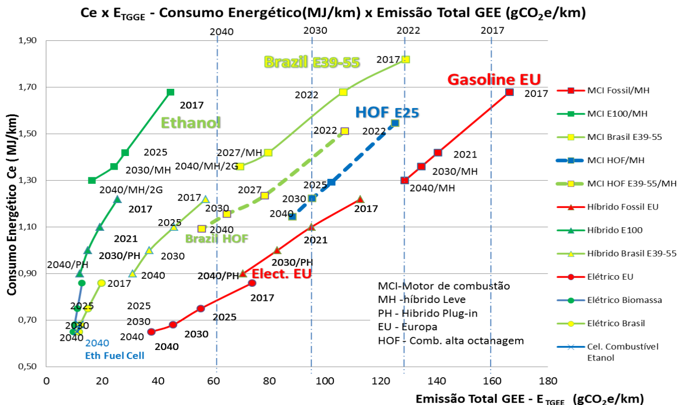
Figura 3 – Ce x E TGEE = Consumo energético x Emissão de GEE poço à roda por quilômetro.
