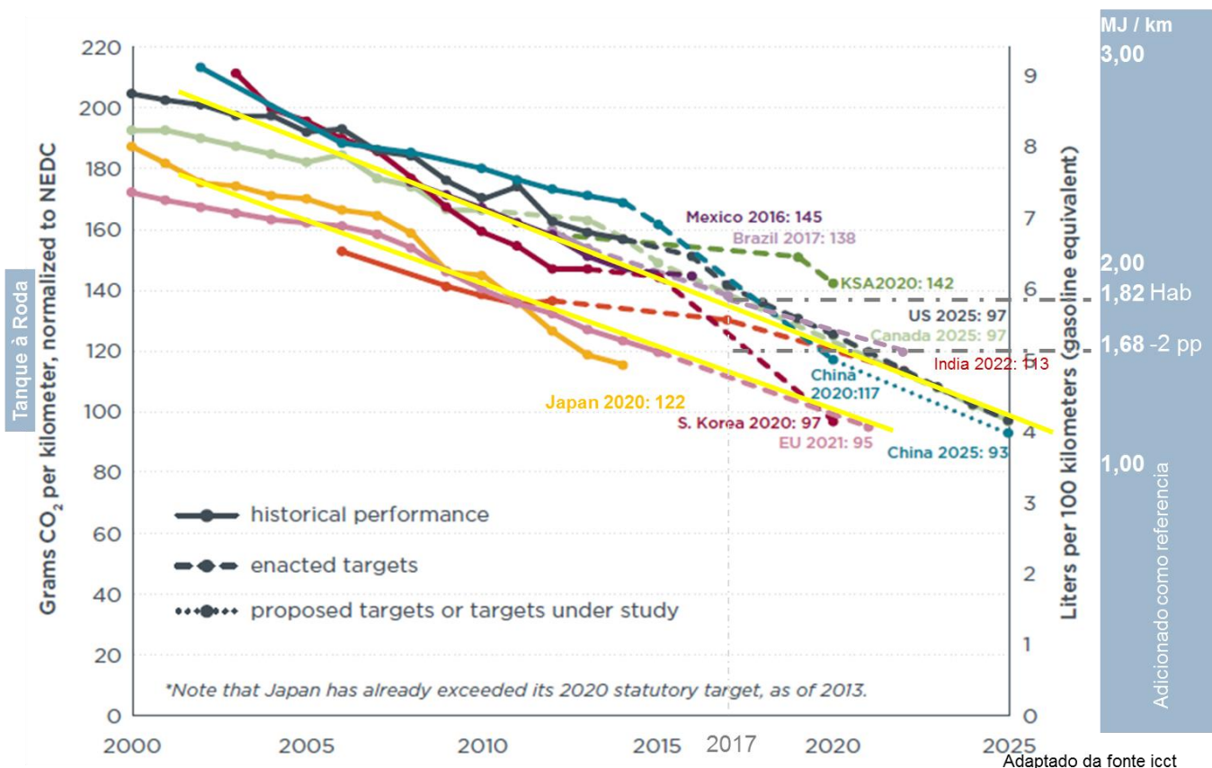
Figura 4 – Evolução dos Limites de Eficiência Energética.
